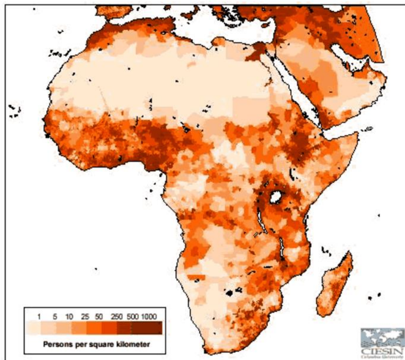
Afrika népsűrűsége
